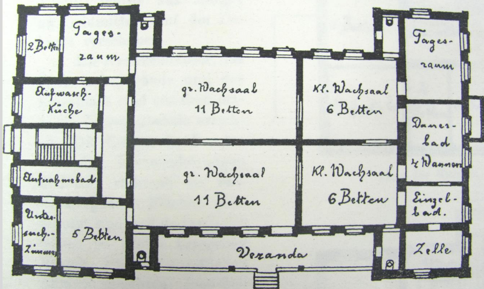
Haus für Unruhige. — Grundriß.
